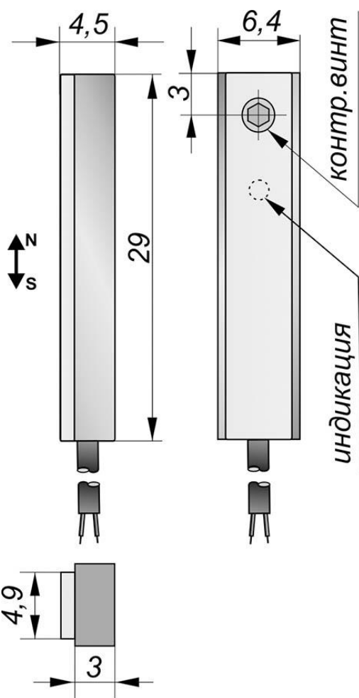
Габаритный чертеж
