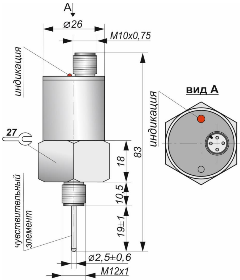
Габаритный чертеж
