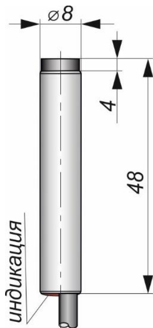
Габаритный чертеж
