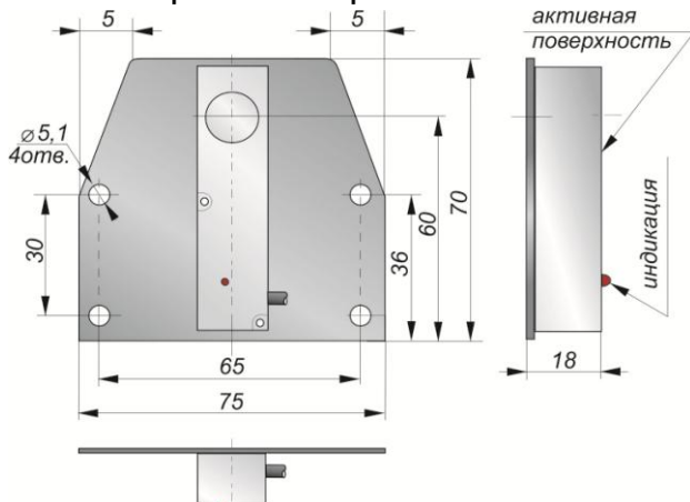
Габаритный чертеж
