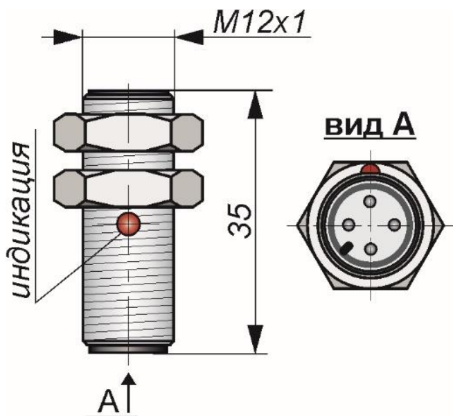
Габаритный чертеж
