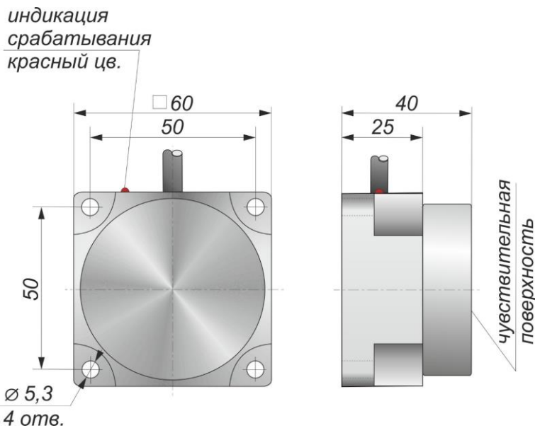
Габаритный чертеж
