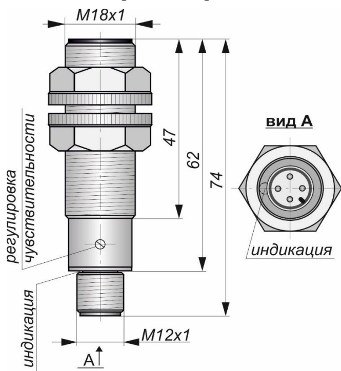
Габаритный чертеж
