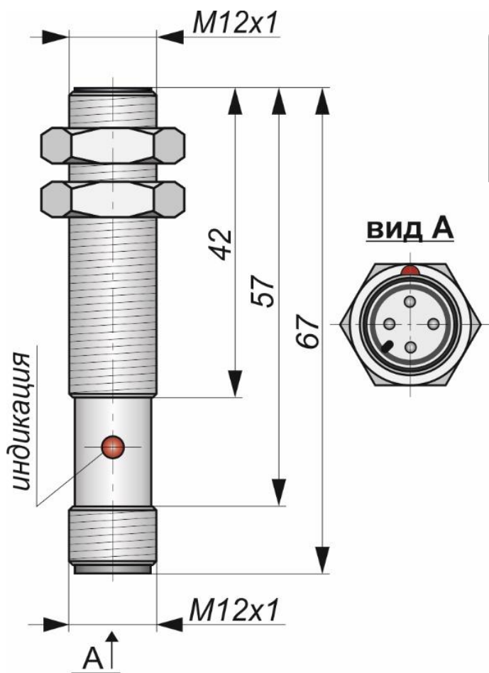
Габаритный чертеж
