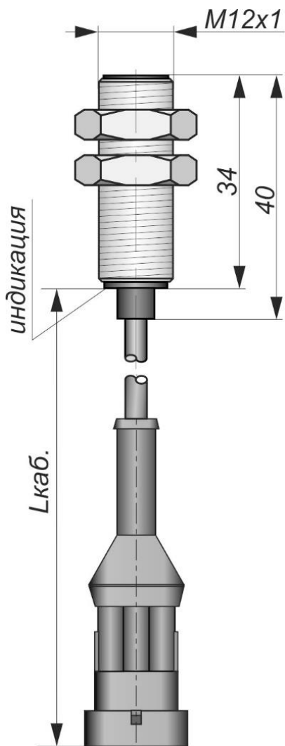
Габаритный чертеж
