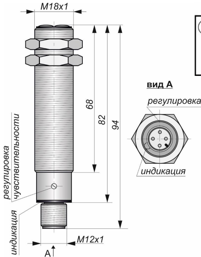
Габаритный чертеж
