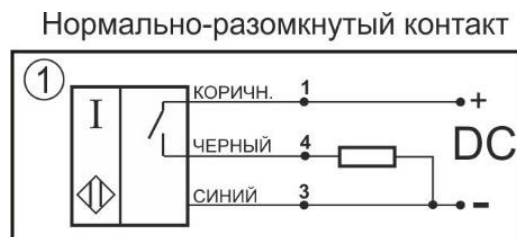
Схема соединения
