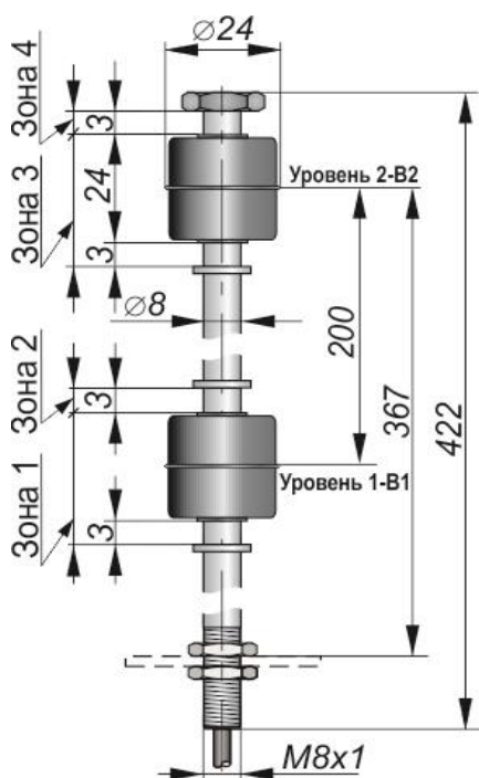
Габаритный чертеж
