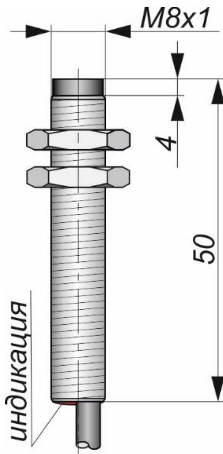
Габаритный чертеж
