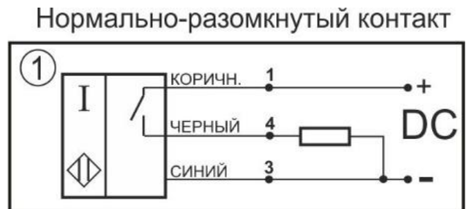
Схема соединения
